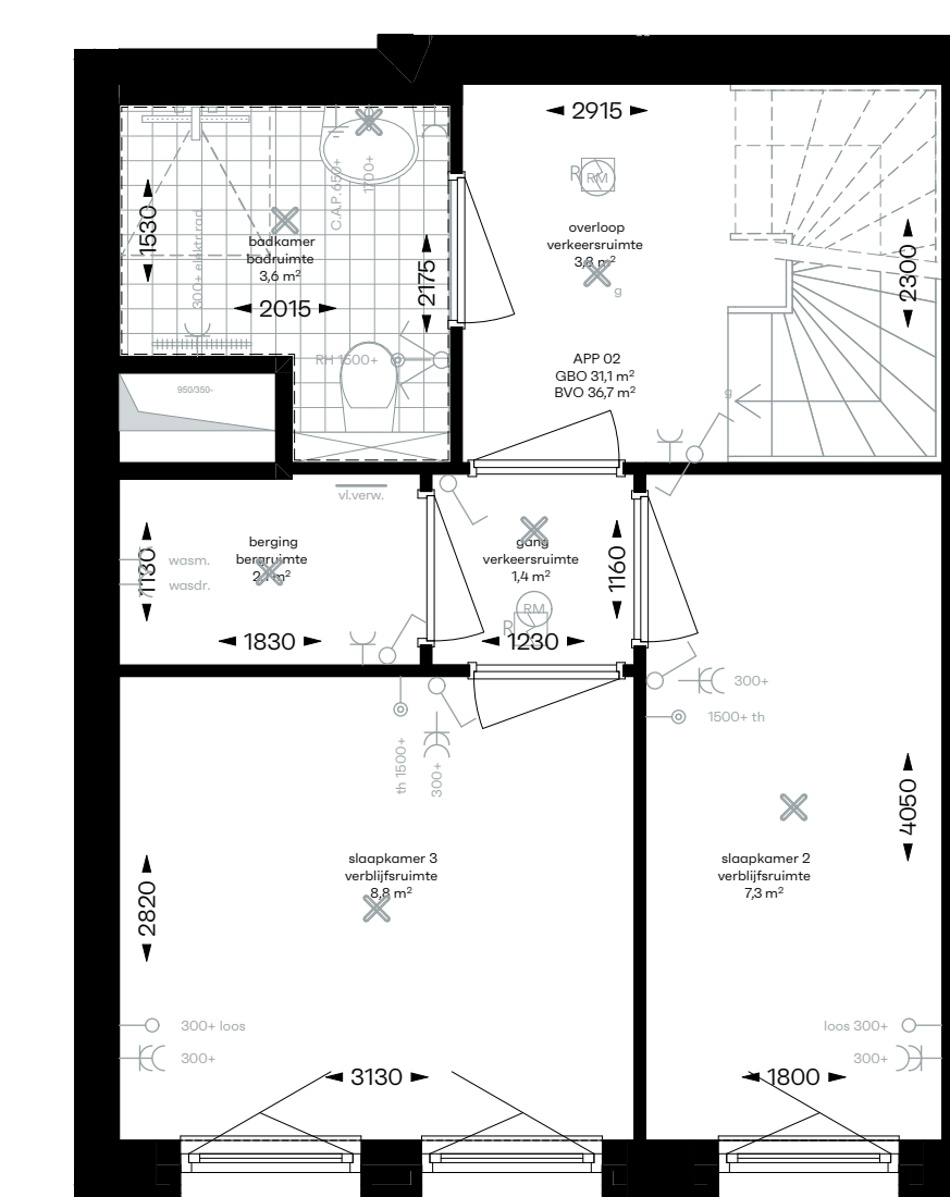
1:50 1e verdieping
